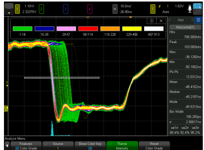
Рисунок 15. Градации цвета и гистограмма для фронта синхриимпульса, подверженного джиттеру.
