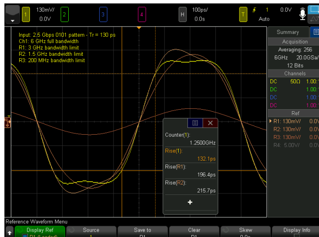
Рисунок 1. Измерение времени нарастания фронта длительностью 130 пс (от 10% до 90%). Результаты измерения времени нарастания:
